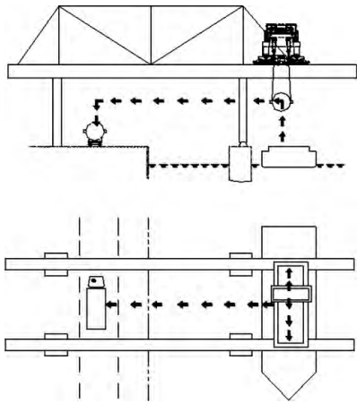
图 3 悬臂钢结构基础的移动式桥吊装卸工艺
