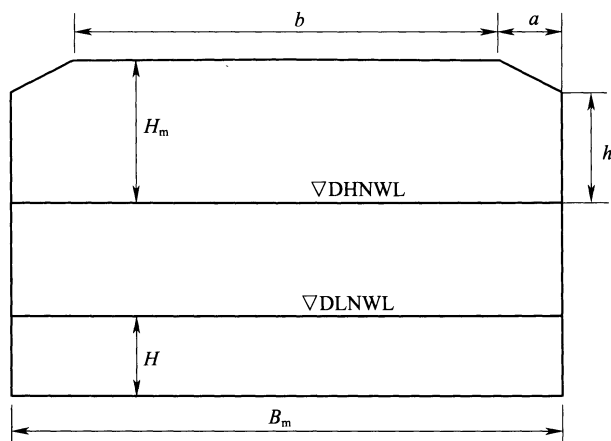
图 5.2.2 通航净空示意图
