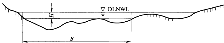
图 3.0.2 天然和渠化河流航道横断面图
