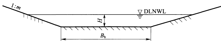
图 3.0.3 限制性航道横断面图
